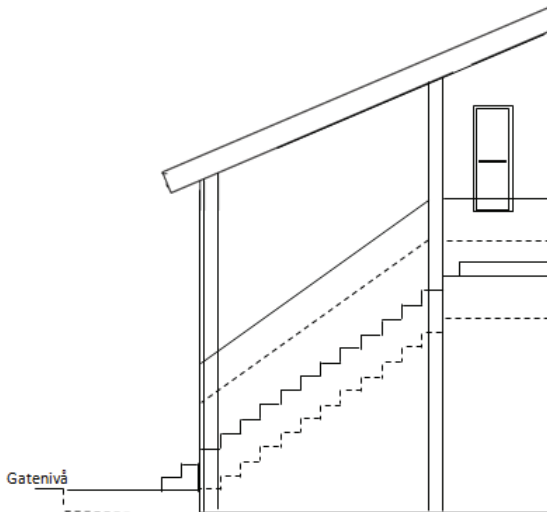
Figur 2 Fasadeendring. Tegningen viser plassering av trapp og rekkverk – før (stiplet) og etter (heltrukken) endring. I dette eksempelet ligger gatenivå like i overkant av nederste trappetrinn.
