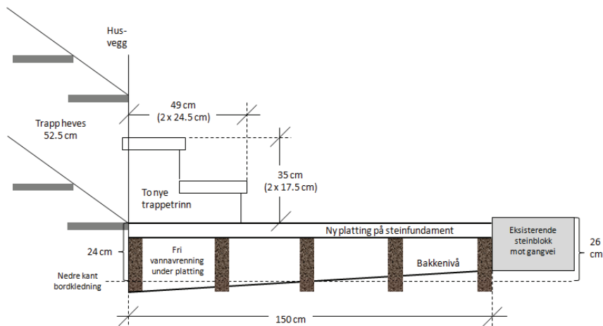
Figur 3 Eksempel på plattung og ekstra trappetrinn mellom trapp og gangvei.
