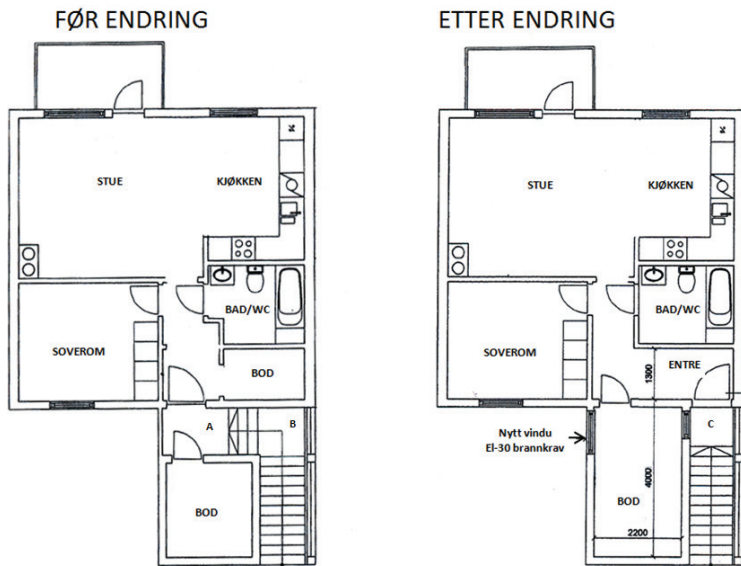
Figur 1 Planløsning før og etter endring. Høydeforskjellen mellom plattform A og B er ca 78 cm.
